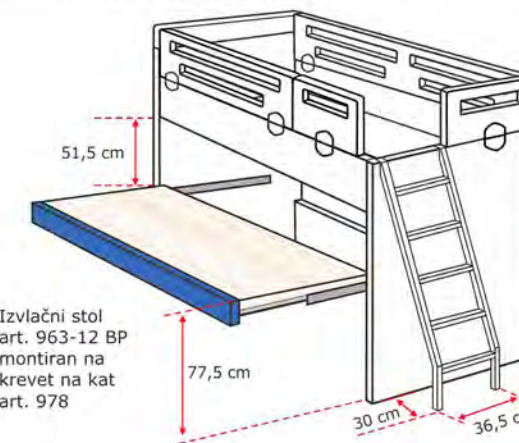
Krevet na kat art. 978-12 dim. š.96 x v.175 x d.205 cm Za madrace dim: 200 x 90 cm
