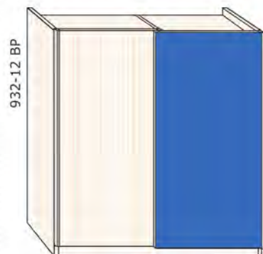
Ormar dvokrilni klizni art. 932-12 š.198 x v.225 x d.63,5 cm
