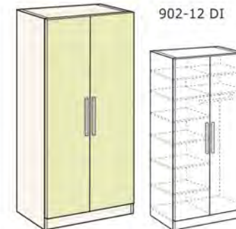
Ormar dvokrilni art. 902-12 š.100 x v.219 x d.60 cm
